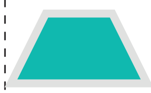
Trapezium
